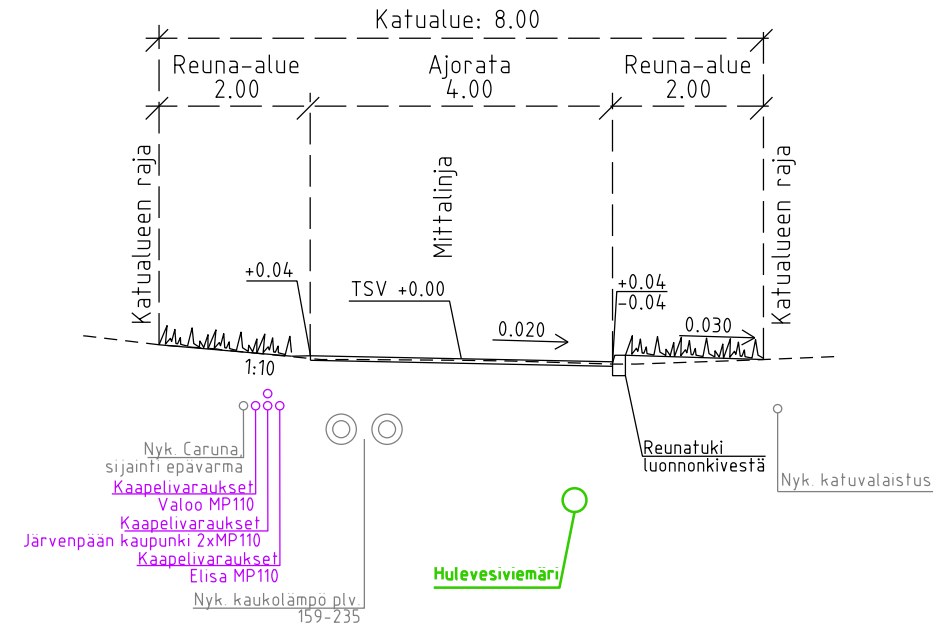
Mailaskuja Tyyppi-poikkileikkaus plv 7-85, 159-235 (pl 75) 1:100
