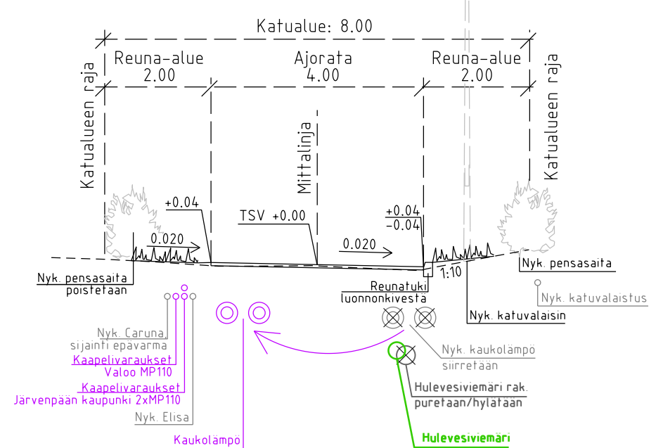
Mailaskuja Tyyppi-poikkileikkaus plv 92-151 (pl 140) 1:100
